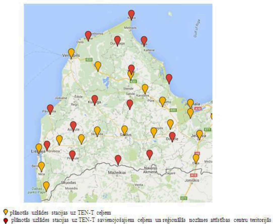
17.attēls. Potenciāli iespējamais Latvijas nacionālais ETL ātrās uzlādes tīkla ģeogrāfiskais izvietojums Kurzēmē 11
