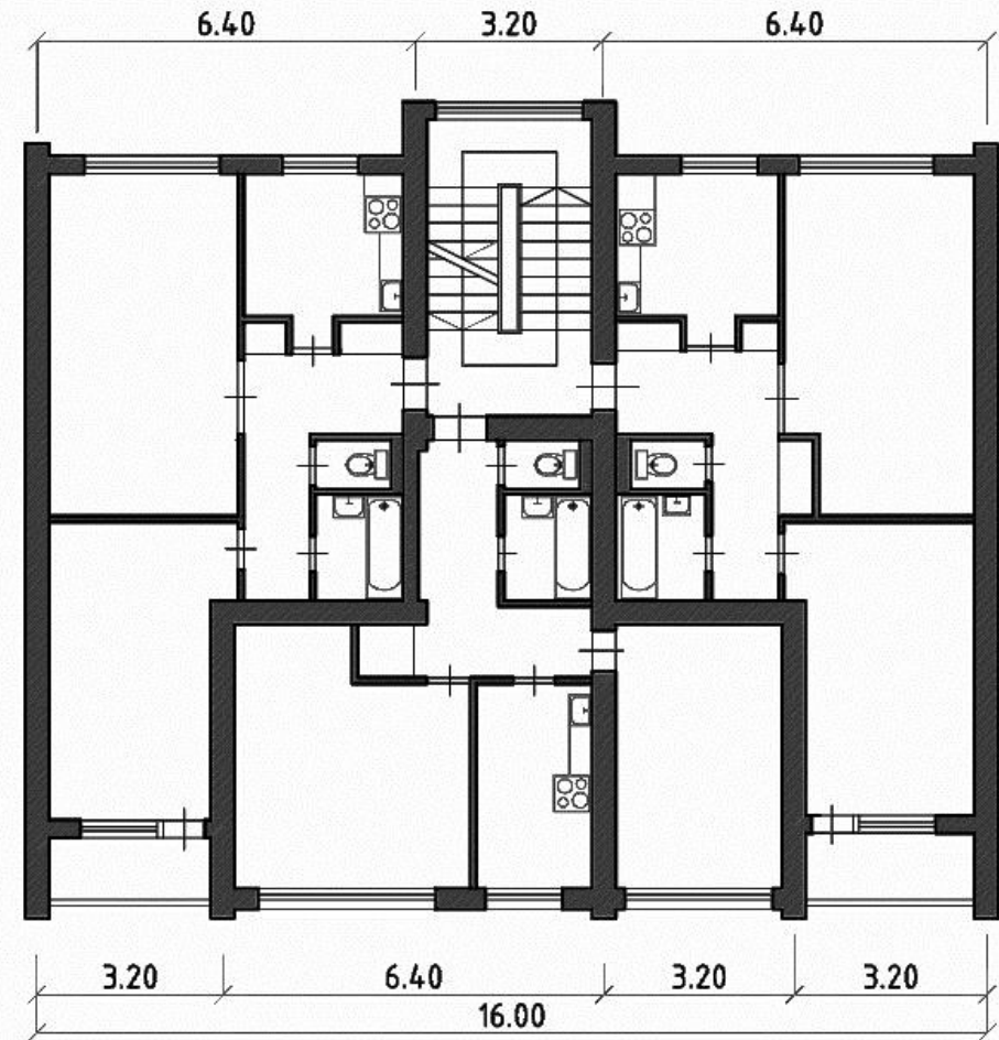
SEKCIJA 2-2-2
